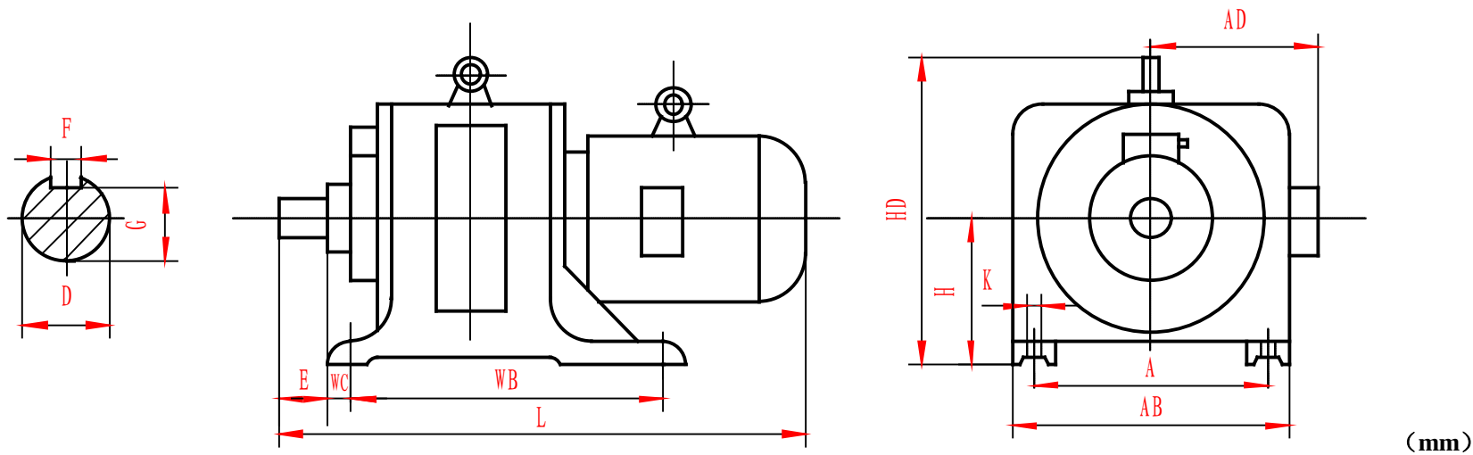
YCT 系列电磁调速电动机外形及安装尺寸
